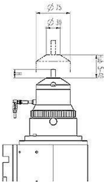
Ansicht B
